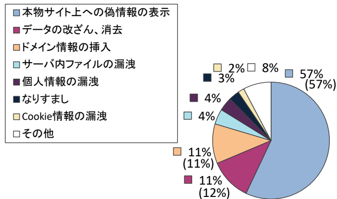
図2-17. 届出累計の脆弱性がもたらす影響別割合
